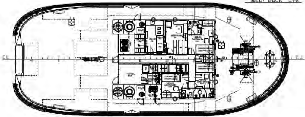
MAIN DECK 主甲板
