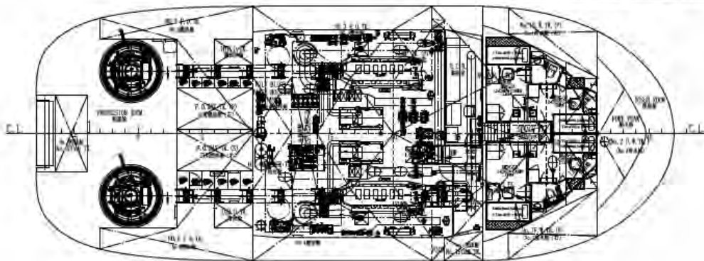
BELOW MAIN DECK 主甲板下
